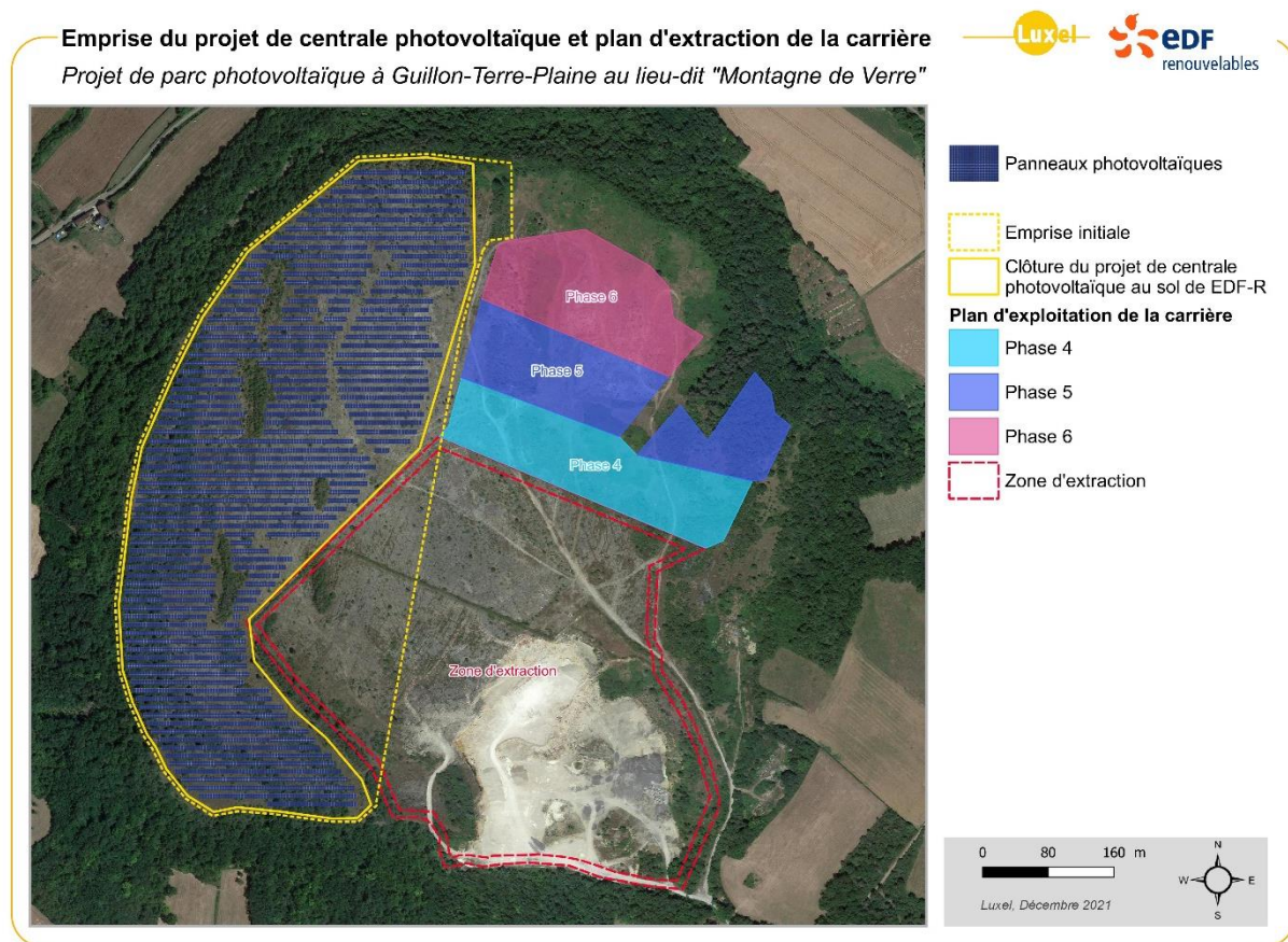
Figure 7 : Emprise du projet et plan d'extraction de la carrière
