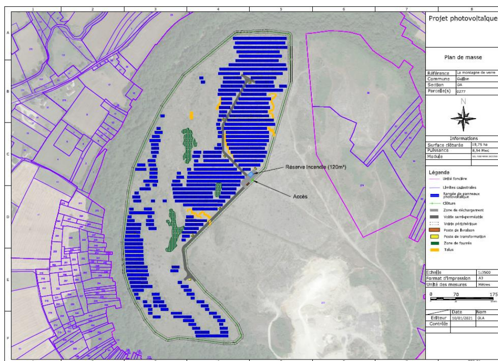
Figure 6 : Plan d'implantation de la seconde variante (Scénario 5)
