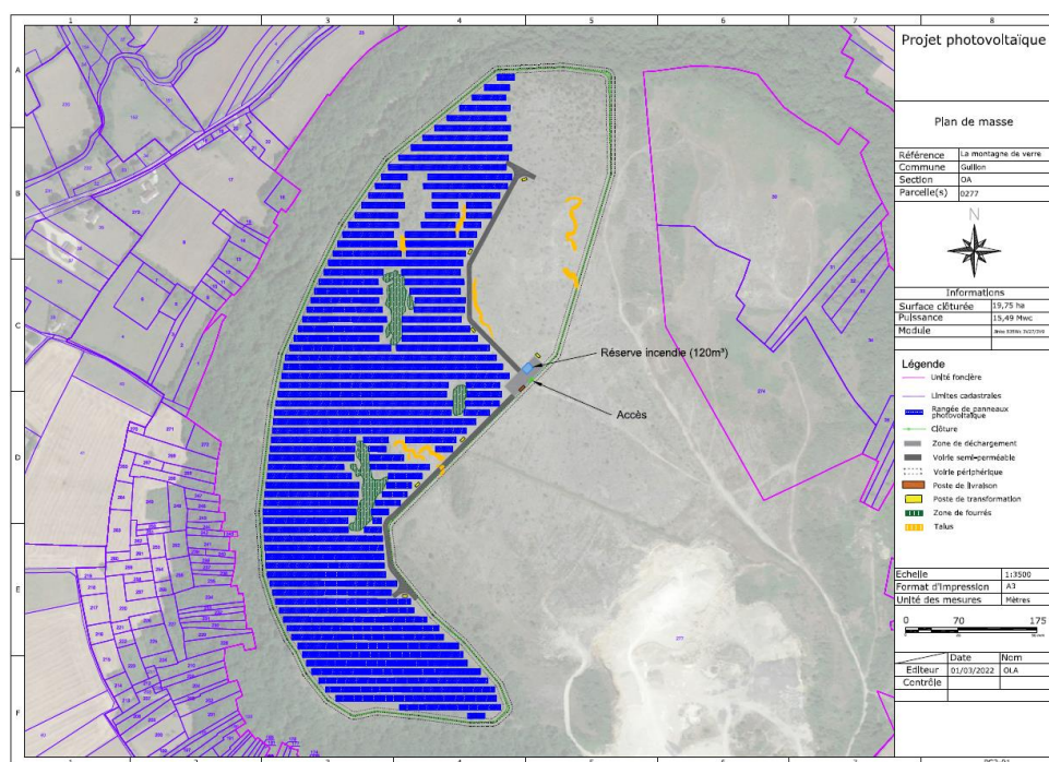
Figure 5 : Plan d'implantation de la première variante (Scénario 4)
